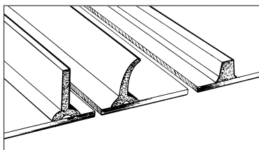
Påvulkade medbringare
